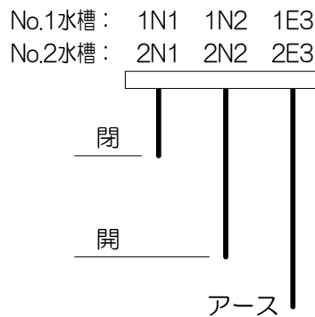
図7-3 電磁弁自動制御用電極について
